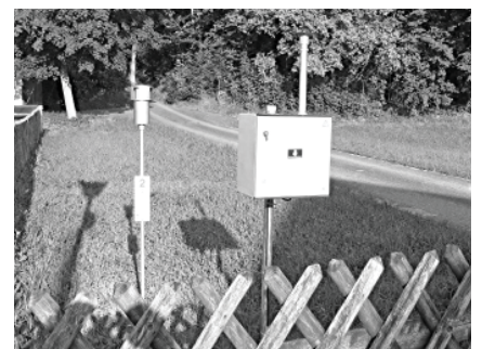
Messstation an der Waxensteinstraße - rechts im Bild der elektronisch betriebene Mini-Volumensammler für den Feinstaub und links im Bild der Sedimentationssammler für den Grobstaubanteile in der Luft
